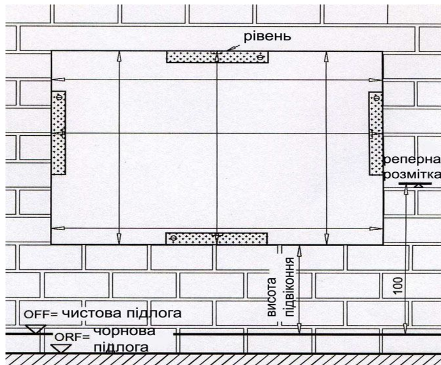
Рисунок 3 – Схема обмірювання віконного прорізу
