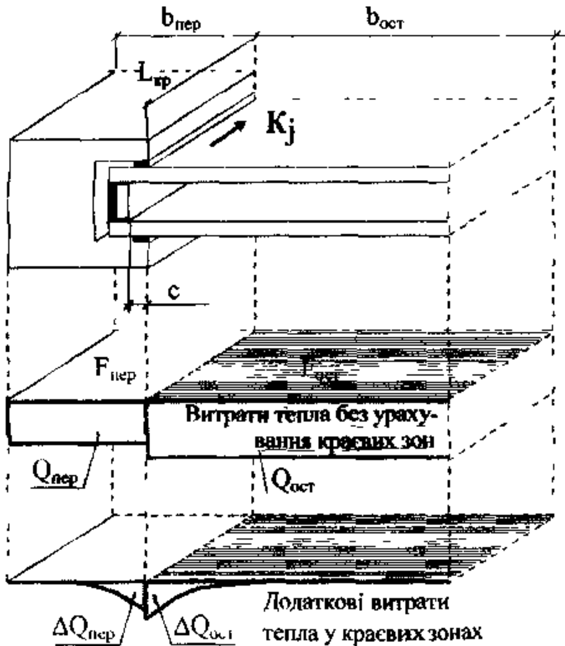
Рисунок К.1 Схема розподілення теплових потоків скрізь остеклення та непрозору частину віконних блоків з урахуванням краєвих зон
