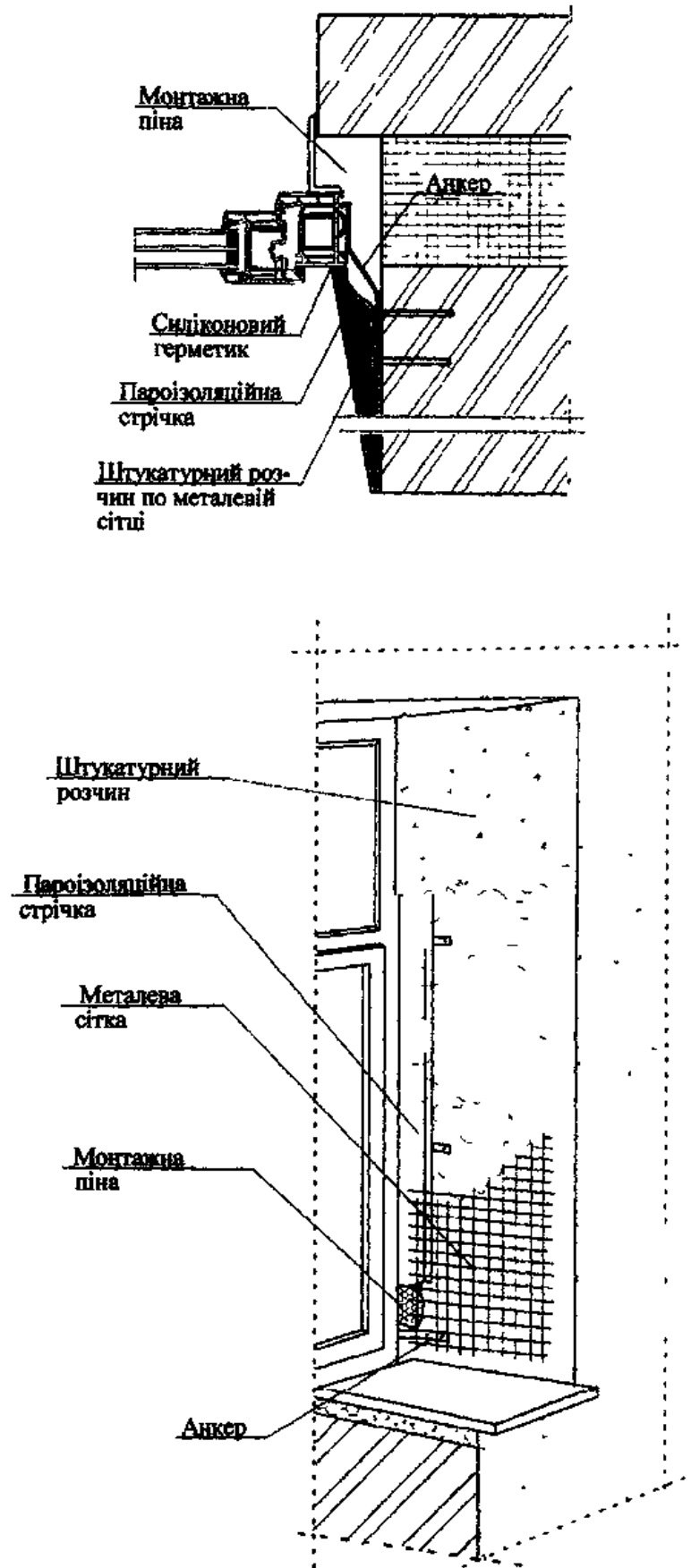
Рисунок 23 – Конструктивні особливості облицювання віконних укосів штукатурним розчином у тришарових стінових панелях з утеплювачем
